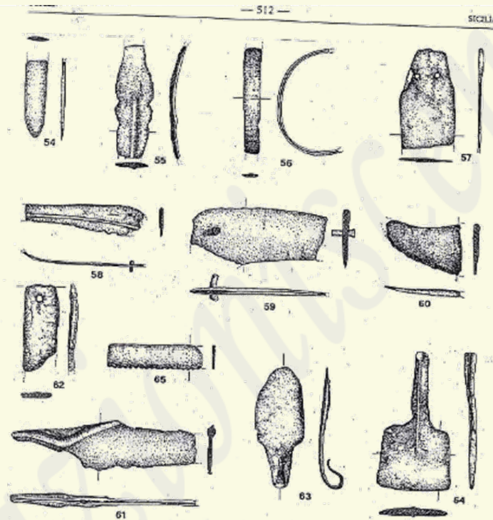
Fig. 18. - Pugnaletti (nn. 54-56), pugnale (n. 57), coltelli (nn. 58-62), rasoio (n. 63), sgorbis o palette (n. 64), sega (n. 65) (1:2).
